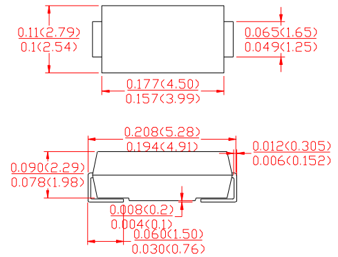
SMA(DO-214AC)
